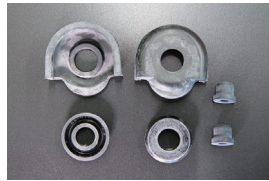
リヤホイールシリンダーカップキット
