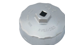
カップ型オイルフィルターレンチ 品番：AVSA-080 適合：18RG 価格：¥2,890 ※フィルター直径 80φ
