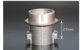
A12 クラッチスリーブ (27mm) ¥1,900 ■適合 A12標準品 A14,A15にクロモリ軽量フライホイール を装着した時に交換必要。
