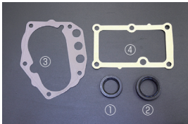
71C, 71B パッキン&シール ①フロントオイルシール ¥280 ②リアオイルシール ¥430 ③フロントカバーパッキン ¥990 ④71Cシフトハウジングパッキン (R32タイプ¥470 シルビア¥830)
