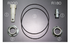
R200/R180 デフパーツ R200 R180 ①プリーザー ¥310 ¥280 ②ピニオンロックナット ¥1,490 ¥350 ③リテーナーOリングSET — ¥540
