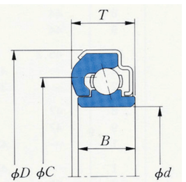
日産クラッチリリースベアリング 品番: 40751S ¥1,910 ■適合 (標準) L6 A型 FJ20 ※サイズ D=74.5 d=40 T=19 B=17 C=62
