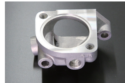
L型 STD サーモハウジング 適合：ワンキャブ、SUキャブ車 車種：S30,GC10,GC110,KHC130 価格：¥2,770 *1/4サイズの水の取り出し口あり
