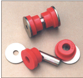
S30デフキャリアブッシュSET
