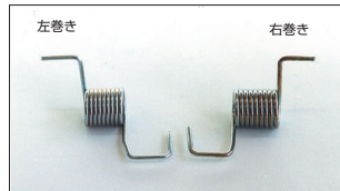
●リターン Springs ¥700 スロットルの戻り側の Springsでエンジン型式によって右巻きと左巻きがあり。
