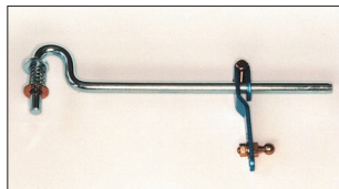
●L6ジョイント (アルミ押しレバー付き) ¥8,000 L6ロッド式インマニの構成部品でリンケージをロッドで駆動するためのジョイントパーツ。 (2024.11.14 更新)
