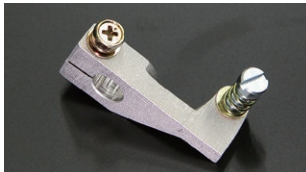
●調整レバー (右向き) ¥1,850 (軸径: 10φ) 押しレバーによるスロットル開度を微調整するときに必要。
