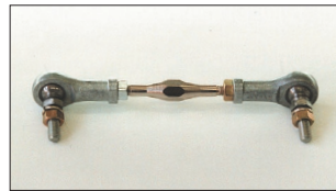
●ターンバックル (両ピロ) ¥4,400 両側にピロボールを使用することで、スポーツ走行に於いてボールジョイントが外れるトラブルを解消。片側が逆ネジでエンジンに付けたまま長さ調整可能。
