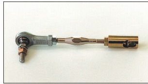
●ターンバックル (片ピロ) ¥3,700 ソレックスの場合はキャブ側のボールが外れないため片ピロタイプをおすすめ。片側が逆ネジでエンジンに付けたまま長さ調整可能。
