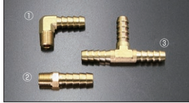
●燃料ホースジョイント (2026.3.16更新) ① 8φ-1/8 L型ジョイント 本体 ¥1,000 ② 8φ-1/8 ストレートジョイント 本体 ¥600 ③ 8φ-T型ジョイント 本体 ¥2,200
