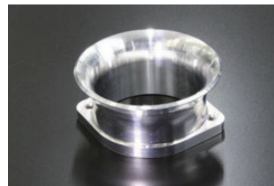
●SOLEX 50φ 35mmエアファンネル ・品番 F-S5035 ¥7,500 ※アルミ削りだし品 (内径53)
