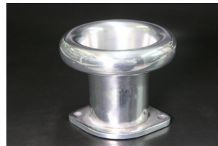
●40φ 70mm カールファンネル ・適合 SOLEX40φ WEBER40φ ¥5,000 ・品番 CF-4070 (内径40)
