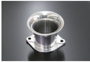
●40φ 50mm エアファンネル (STD) ・適合 SOLEX40φ WEBER40φ ¥5,000 (2026.3.16更新) ・品番 F-4050S (内径40)
