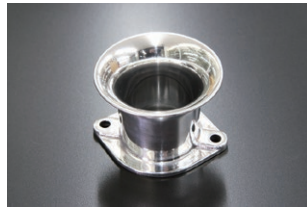
●40φ 50mm エアファンネル (ポリッシュ) ・適合 SOLEX40φ WEBER40φ ¥6,000 (2026.3.16更新) ・品番 F-4050P (内径40)
