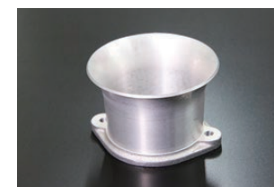
●SOLEX 50φ 50mmエアファンネル ・品番 F-S5050 ¥8,500 (2026.3.16更新) ※アルミ鋳造加工品 (ミクニ純正仕様: 内径53)
