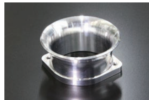
●SOLEX 50φ 35mmエアファンネル ・品番 F-S5035 (2026.3.16更新) ※アルミ削りだし品 (内径53) ¥8,500
