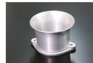
●SOLEX 50φ 50mmエアファンネル ・品番 F-S5050 (2026.3.16更新) ※アルミ鋳造加工品 (ミクニ純正仕様: 内径53) ¥8,500
