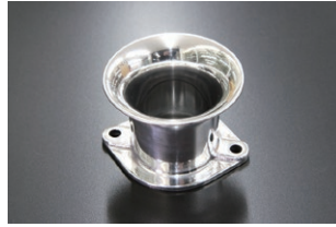
●40φ 50mm エアファンネル (ポリッシュ) ・適合 SOLEX40φ WEBER40φ (2026.3.16更新) ・品番 F-4050P (内径40) ¥6,000
