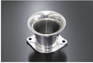
●40φ 50mm エアファンネル (STD) ・適合 SOLEX40φ WEBER40φ (2026.3.16更新) ・品番 F-4050S (内径40) ¥5,000
