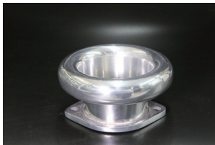
●44-48φ 45mm カールファンネル ・適合 SOLEX44φ WEBER45φ/イタリー製48φ OER45/47φ (2026.3.16更新) ・品番 CF-4445 (内径48) ¥5,000
