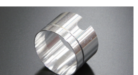
●SOLEX 40φ アウターベンチュリー 品番: N121015 (アルミ削り出し品) サイズ: 30φ 32φ 34φ 36φ 37φ 本体 ¥4,000 ※MIKUNI名称: ラージベンチュリー
