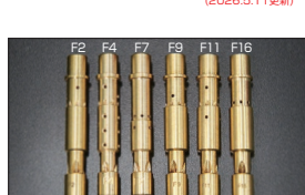
●WEBER エマルジョンチューブ F2 本体 ¥4,500 F2 本体 ¥3,500 F4 本体 ¥4,500 F9 本体 ¥3,500 F7 本体 ¥4,500 F11 本体 ¥3,500 F16 本体 ¥3,500
