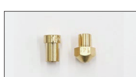
●WEBER ジェット メインジェット#100~#230(#5とび) 本体 ¥600 メインジェット#235~#260(#5とび) 本体 ¥600 エアージェット#100~#230(#5とび) 本体 ¥600 エアージェット#235~#260(#5とび) 本体 ¥600
