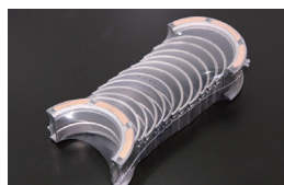
L6 純正0.25アンダーメインメタルSET 原動機： L20,L24,L28 適合：ジャーナルが0.25アンダーで スラストがSTDタイプ 価格： ¥15,700
