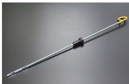
S130 オイルレベルゲージ ※上部からHまでの距離179mm HからLまで19mm 価格： ¥670
