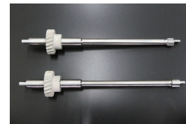
L6 スピンドルギヤ ●後期型：KAMEARI製品 写真上 価格： ¥20,000 (2025.1.1更新) ●前期型：日産純正部品 写真下 価格： ¥20,000 (2024.10.1更新)
