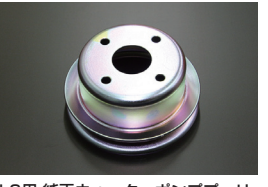
L6用 純正ウォーターポンププリー 原動機：L20~L28 適合：外径116φ 13mmベルト用 価格：¥5,620
