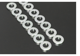
L型 純正ヘッドボルトワッシャーSET 原動機：L20,L24,L28,L14,L16,L18 適合：L型全車 価格：L6 ¥3,080 L4 ¥2,200
