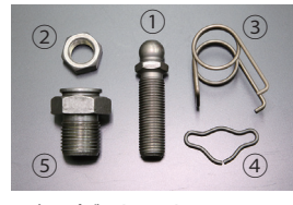
L型用 ビボットセット ¥1,290 /1set (単品) ①ビボットアジャストスクリュー ¥320 ②ビボットロックナット ¥320 ③ロックスプリング ¥120 ④ビボットリテーナー ¥120 ⑤ビボットワッシャー ¥410
