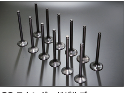
L20 スタンダードバルブ 適合：L20 サイズ：IN:38φ EX:33φ 価格：IN ¥3,000/1本 EX ¥3,000/1本
