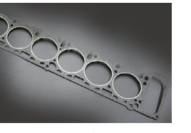
L20 STDヘッドガスケット 適合：L20 車種：GC10~HR30, S30, KC130等 価格：¥5,800 (社外品) ¥18,100 (純正品)
