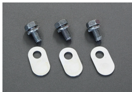
L6 カムホルダーオイルシャワープラグ ¥1,200/SET ・L型前期エンジンにセンター給油カムを装着した時に必要なオイル通路栓。
