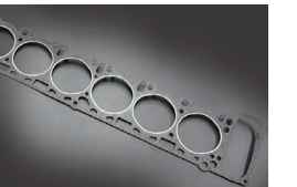
L20 STDヘッドガスケット ■社外品 L20ヘッドG/K ¥5,800 (適合シリンダー：E30 及び Y70) ■日産純正 L20ヘッドG/K ¥19,000 (適合シリンダー：E30 / Y70 / 14S)
