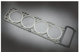
L18 STDヘッドガスケット 適合：L18 車種：510 等 価格：¥4,950 (社外品)
