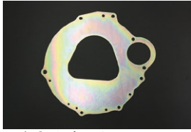
L型 バックプレート (2026.4.6更新) ※S52 マニュアルミッション車用 ¥1,990 (注) ユニクロメッキ (シルバー) に変更されました。
