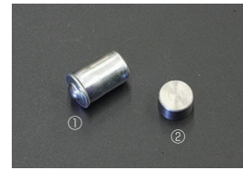
L型 オイルリリーフバルブ&プラグ (2026.4.6更新) ①リリーフバルブ ¥370 ※標準装備品でフィルターの目詰まり時のリリーフ回路/バルブ ②リリーフプラグ ¥800 ※高油圧高回転でもリリーフせず、確実にフィルターを過す
