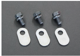
L6 カムホルダーオイルシャワープラグ (2026.4.6更新) ¥1,500/SET ・L型前期型エンジンにセンター給油カムを装着した時に必要なオイル通路栓。
