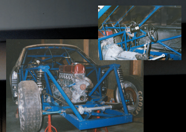
自社製作によるS130ドラッグマシン
