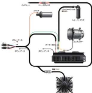
★クーラー配線図
