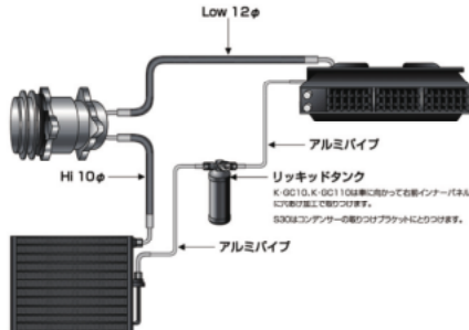
★クーラー配管図
