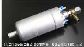
(入口12φ出口8φ 90度向き 52φ全長180mm) ●2.9Lポッシュフューエルポンプ ¥39,000 *吐出量 2.9L/分 (L30~L32レース用) *大容量フューエルレギュレーター2個と8mmリターンパイプ2本で燃圧制御可能
