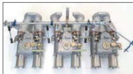
●L28 WEBER45φキット 45DCOE-152キット 本体 ¥220,000 45DCOE-9キット 本体 ¥250,000 ※45φインマニ、インマニG/K、フューエルホース ホースバンド、インシュレーター付き
