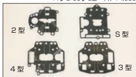
●SOLEX チャンバーカバーガスケット 40φ S型 3型 4型 本体 ¥550 44φ 3型 4型 本体 ¥550 50φ 2型 本体 ¥550
