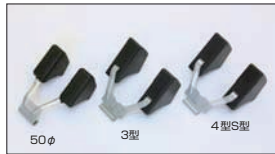
●SOLEX フロート 50φ複製品 ¥13,800 50φ用 製造廃止 3型 製造廃止 4型S型 本体 ¥3,300
