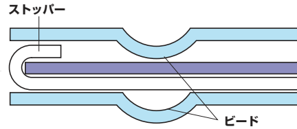
ストッパータイプ断面
