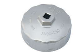
カップ型オイルフィルターレンチ 品番：AVSA-080 適合：18RG 価格：¥2,890 ※フィルター直径 80.5φ
