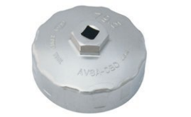
カップ型オイルフィルターレンチ 品番：AVSA-080 適合：A12~A15, U20, H20 価格：¥2,890 ※フィルター直径 80.5φ
