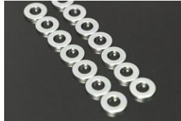
L型 純正ヘッドボルトワッシャーSET 原動機：L20,L24,L28,L14,L16,L18 適合：L型全車 価格：L6 ¥2,940 L4 ¥2,100
