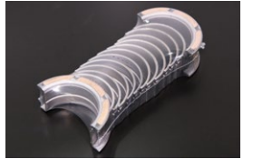
L6 純正0.5アンダーメインメタルSET 原動機：L20,L24,L28 適合：ジャーナルが0.5アンダーで スラストがSTDタイプ 価格： ¥14,000
