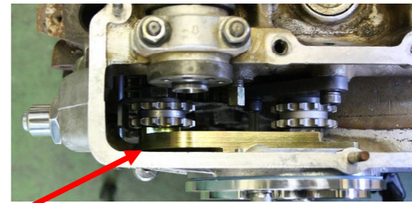
このクリアランスをチェック。特に前期型は干渉する恐れがあります。
