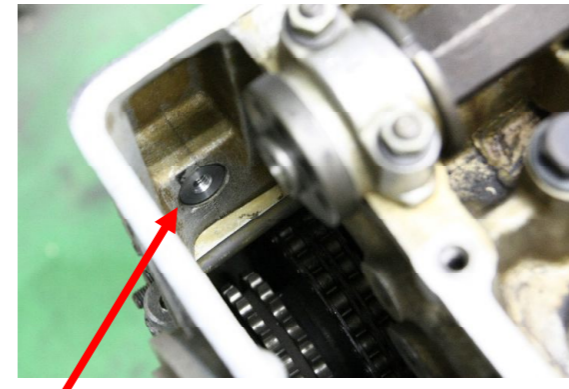
※テンションアジャスターをツライチにする。(パッキンを付けた状態で確認)
