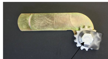
センターボルト締め付けトルク 1100~1200 (N・m) (M12×P1.25 首下 32mm) ※ネジ部にオイル不用
